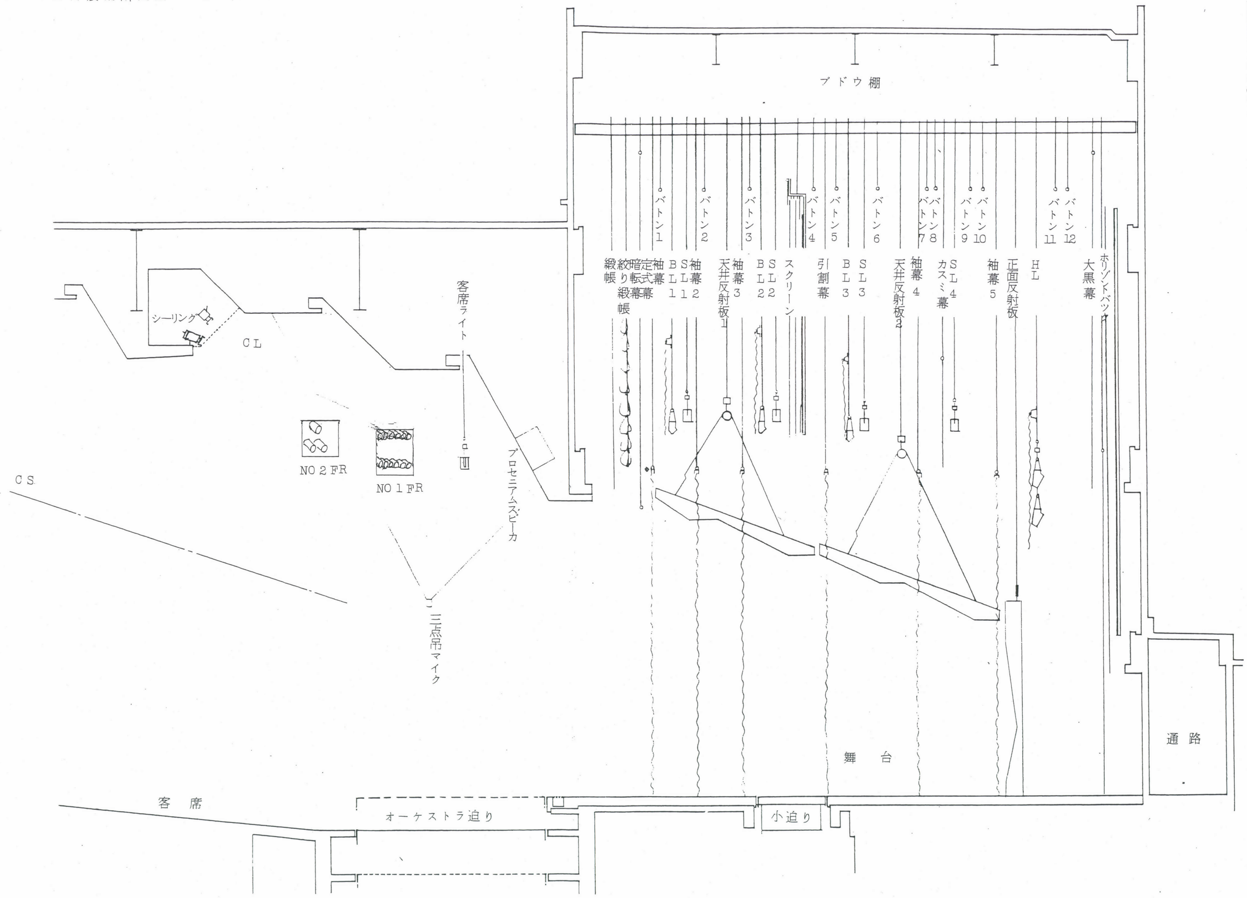
大ホール舞台設備断面図 S = 1 : 100
