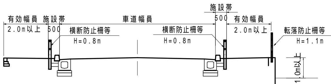
別図 2 1 横断防止柵・転落防止柵の標準横断図 (第 1 7 条第 1 項第 3 号・第 4 号関係)
