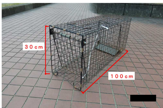
図 1 箱罠詳細 概寸法等
