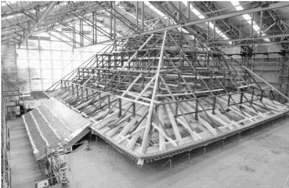
小屋組が組み上がった日向薬師宝城坊本堂
