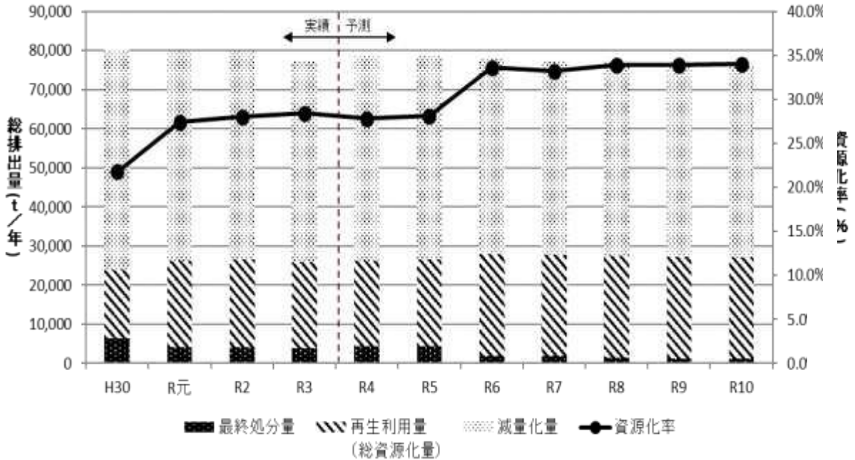
図 1-2 処理処分量等の推移
