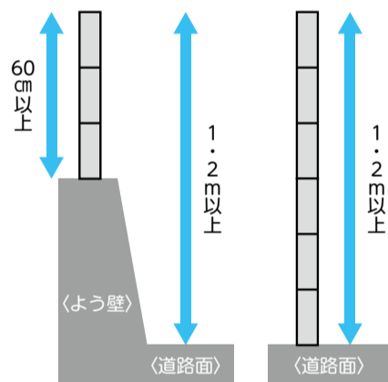
ブロック塀のイメージ図
