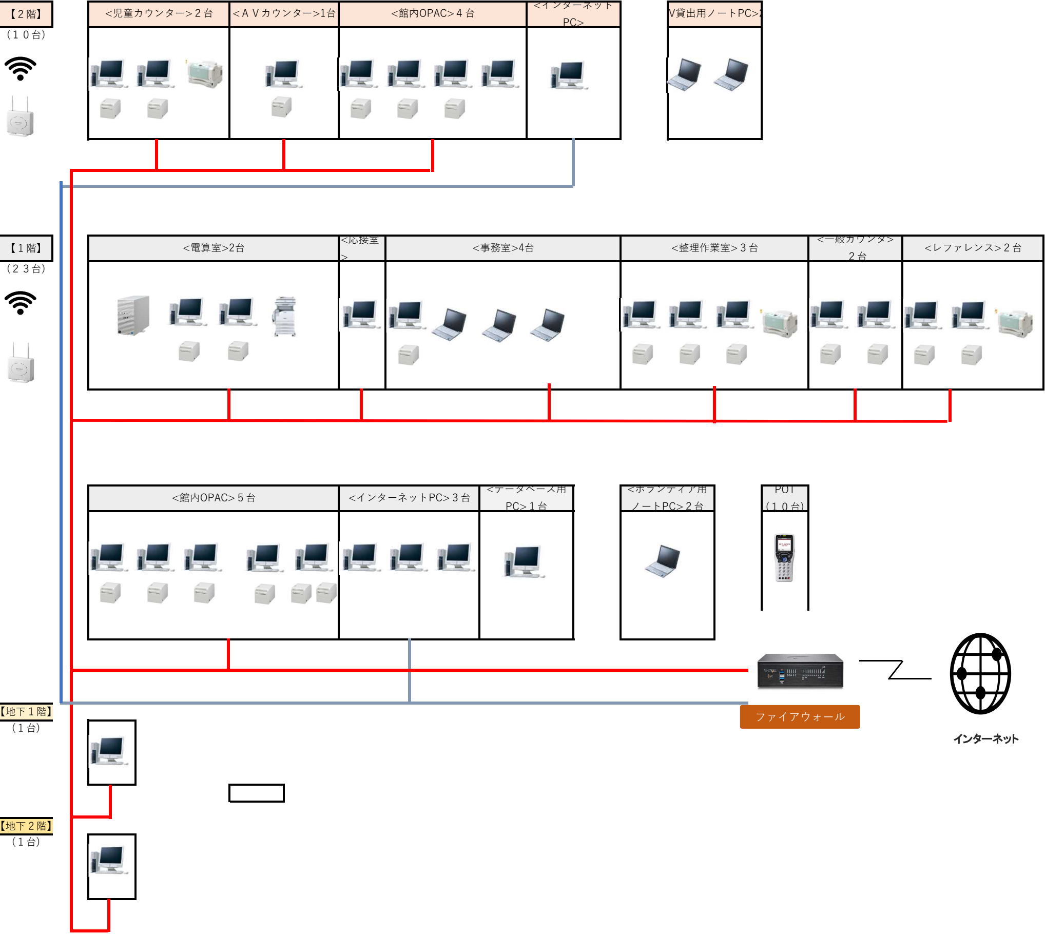
伊勢原市立図書館_システム構成図
